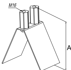
Крепление молниеприемника на конек
