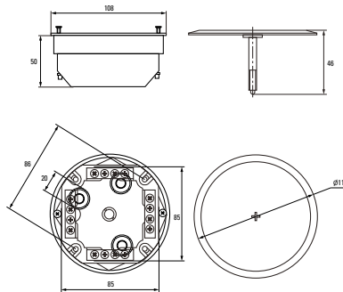
Коробка установочная КМП-020-023
