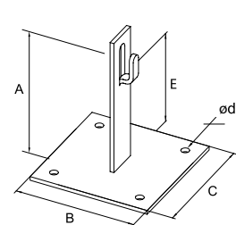
Держатель универсальный L100
