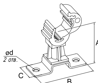
Держатель дистанционный
