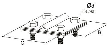
Зажим (полоса-прут) с тремя пластинами
