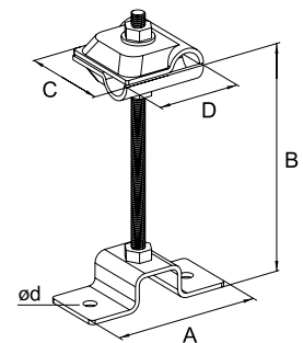
Держатель дистанционный 4x25; 4x30; 4x40; 5x40мм на стене здания
