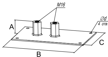
Подставка 1–4 метров
