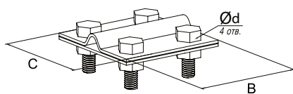
Зажим универсальный (полоса-прут) П-40
