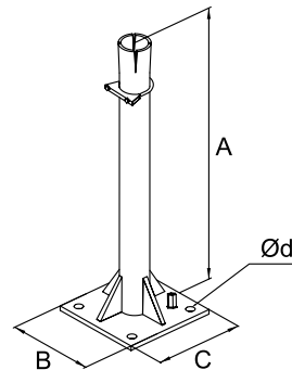
Подставка 5–7 метров
