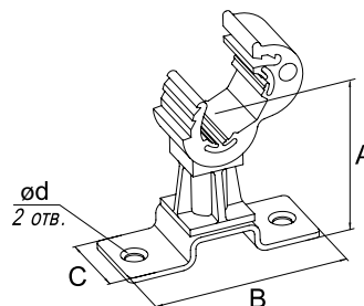
Держатель дистанционный
