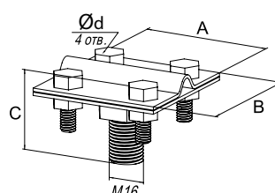
Зажим прута на штыре
