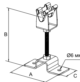
Держатель дистанционный металлический
